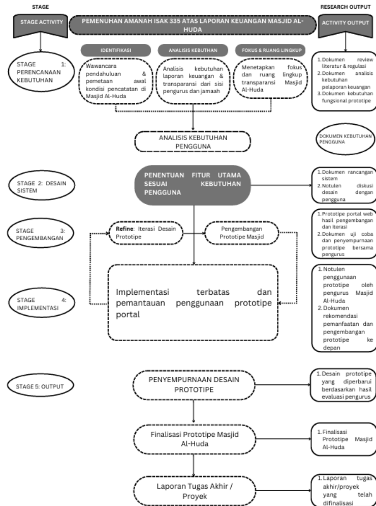
Gambar 3.2 Tahapan RAD
